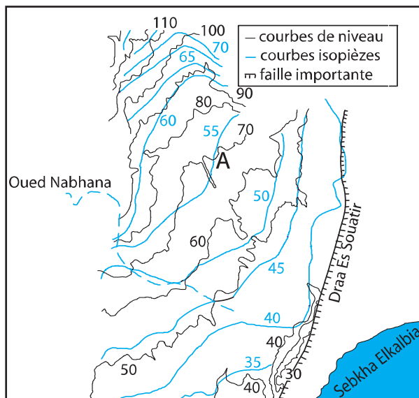
8- Carte piézométrique de la région de Nadhour
