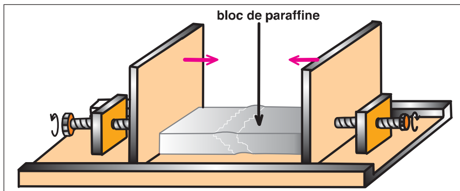
14. Schéma d'un dispositif expérimental permettant de simuler la formation des failles
