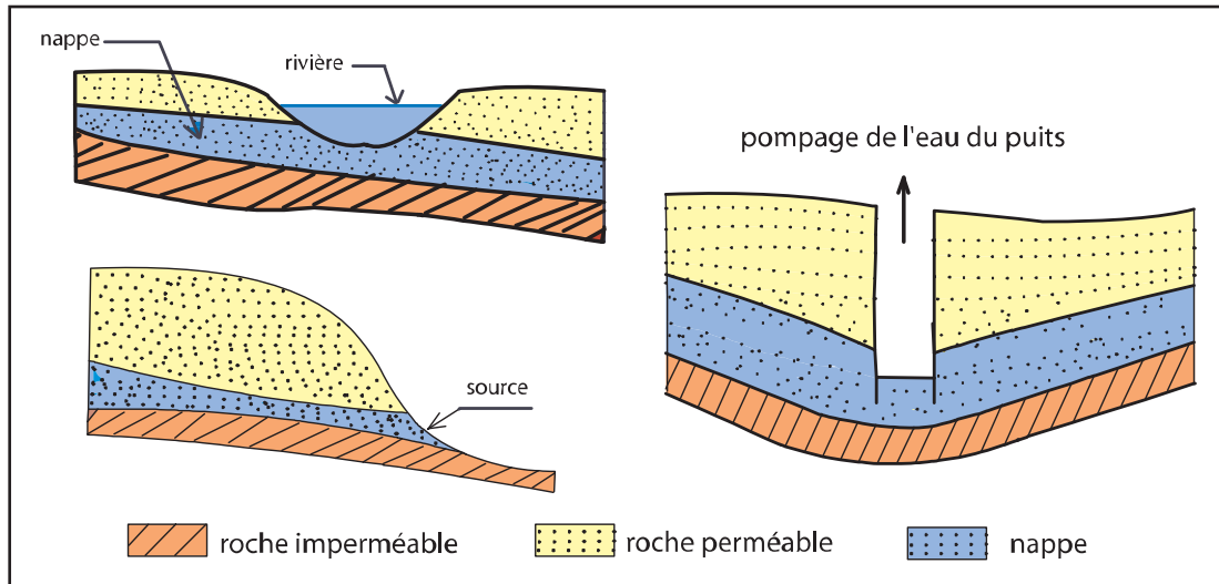
9 - Facteurs de variation de la pression interne de l'eau dans la nappe
