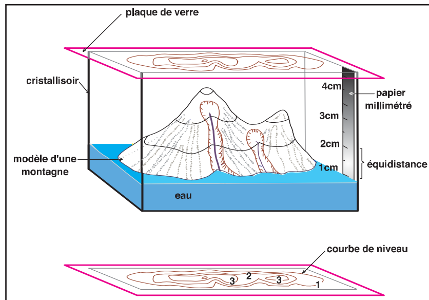
3. Procédé de représentation d'une carte topographique
