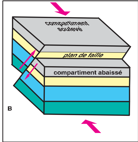
15b. une faille inverse
