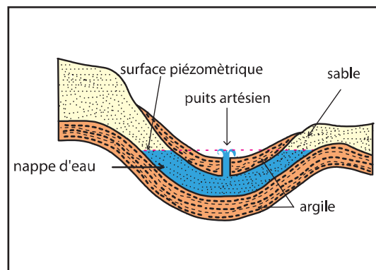
7 b- Coupe géologique montrant une nappe captive.
