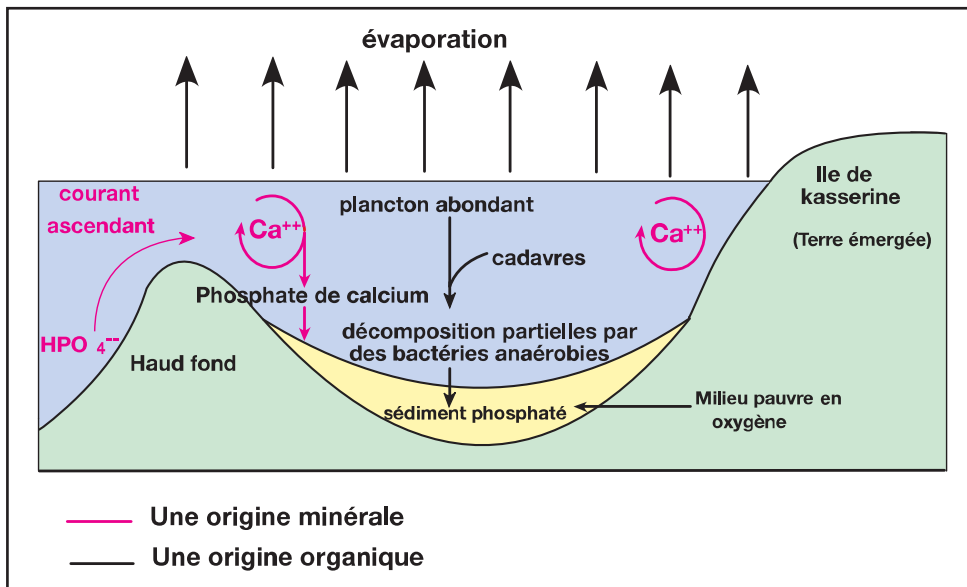
22- Schéma de synthèse de la genèse du phosphate
