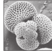
6b. Les globigérines sont des microfossiles de mers chaudes et profondes de l'éocène (ère tertiaire) (Cap Bon, Région de Tunis)
