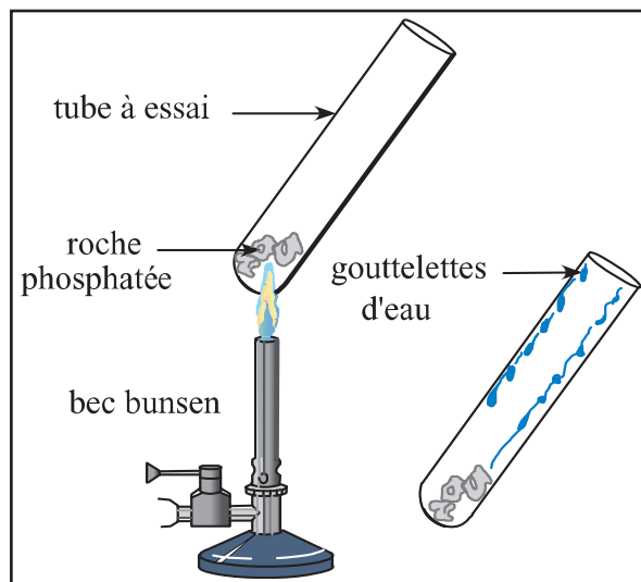
14- Expérience de l'action de la chaleur sur une roche phosphatée
