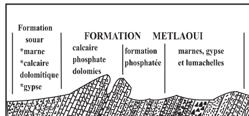
18 - Les affleurements phosphatés à Oued Thelja
