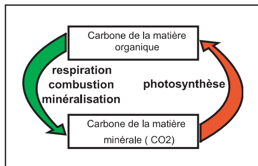
4 -Schéma simplifié du cycle du carbone
