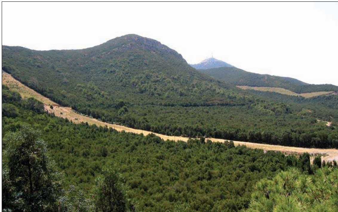
La forêt de Djebel Boukornine : une forêt de Thuya de berbérie
