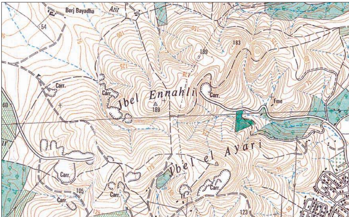
2. Extrait d'une carte topographique de l'Ariana à l'échelle 1/25000
