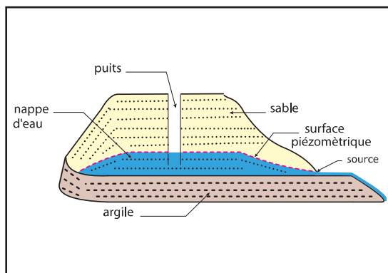
7a- Coupe géologique montrant une nappe libre.
