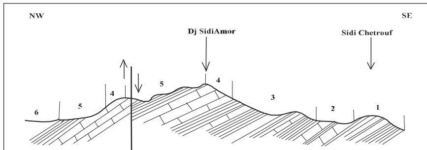
2. Extrait de la carte géologique de l'Ariana (1/50000e) et coupe géologique correspondante (II)
