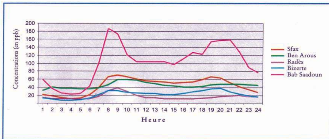
15- Evolution journalière des oxydes d'azote ( \text{NO}\dots ) pour l'année 2003 dans différentes villes
