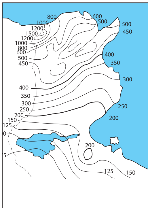
4- Carte des précipitations
