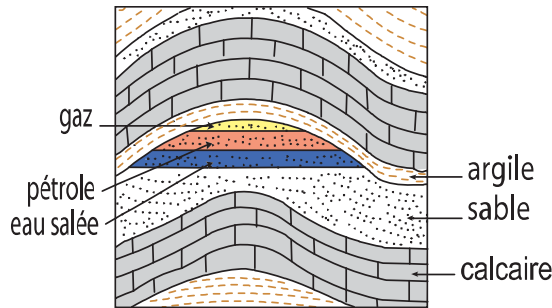
8a- Un anticlinal
