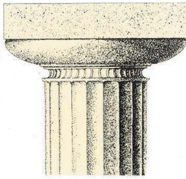
التاج الدوري
