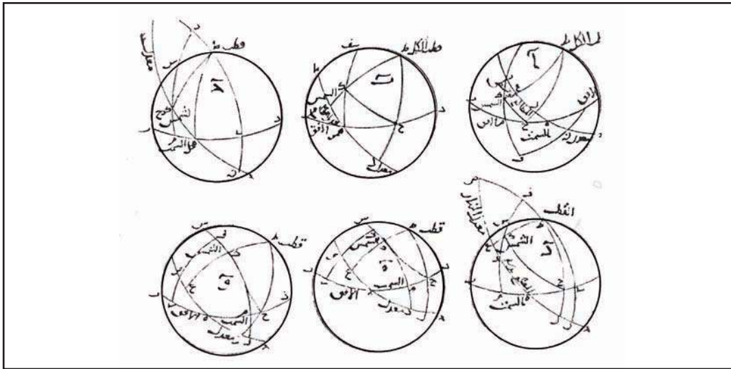
عن مخطوط للبتاني (المتحف البريطاني بلندن) ورد بكتاب «المتع في الأدب» (5 ث ج II الشركة التونسية للتوزيع 1973)
