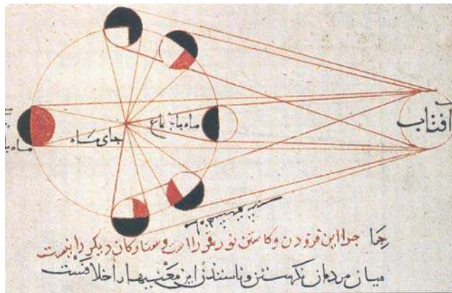
خسوف القمر
