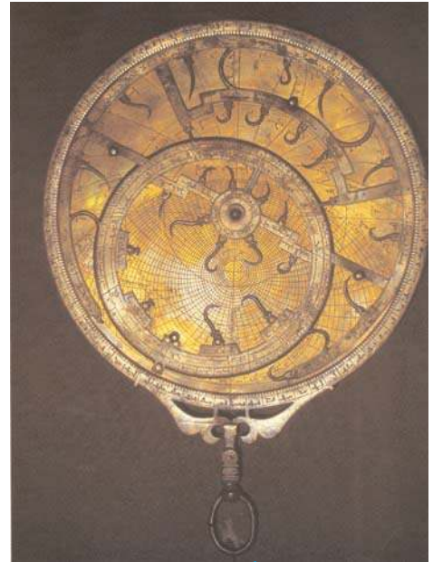
الأسطرلاب
